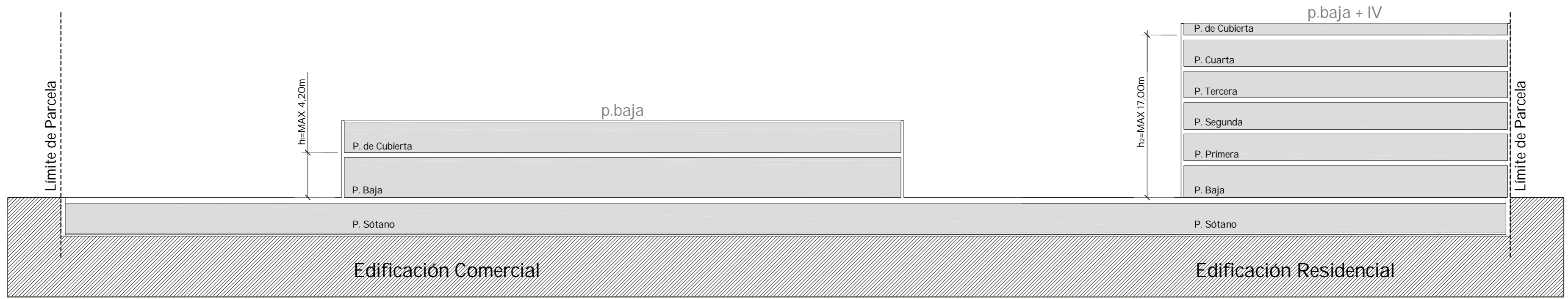
Sección 1 Escala: 1/300
